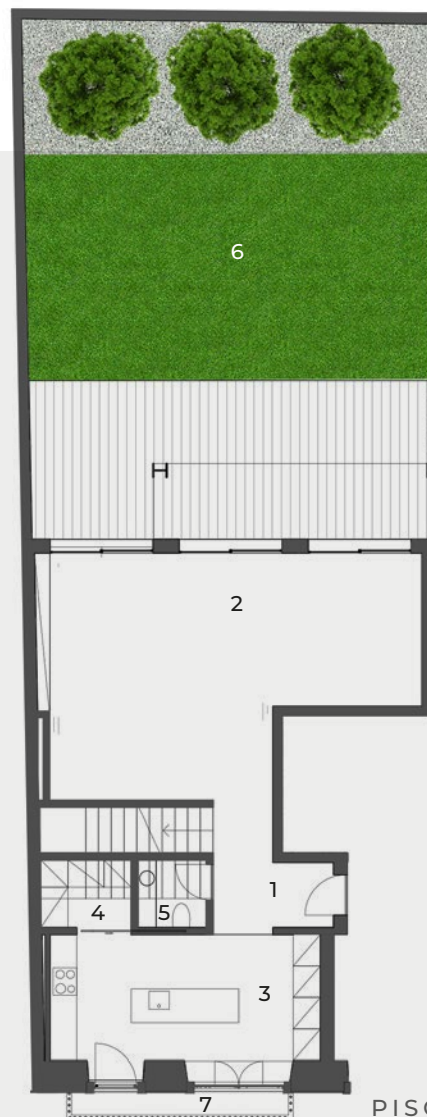
PISO 0
