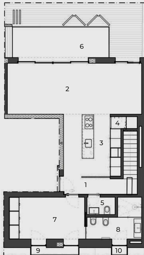
PISO 3
