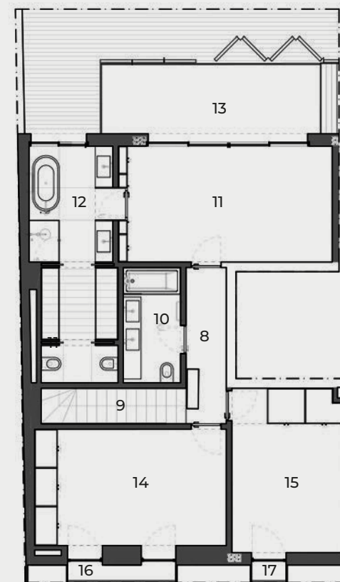
PISO 1
