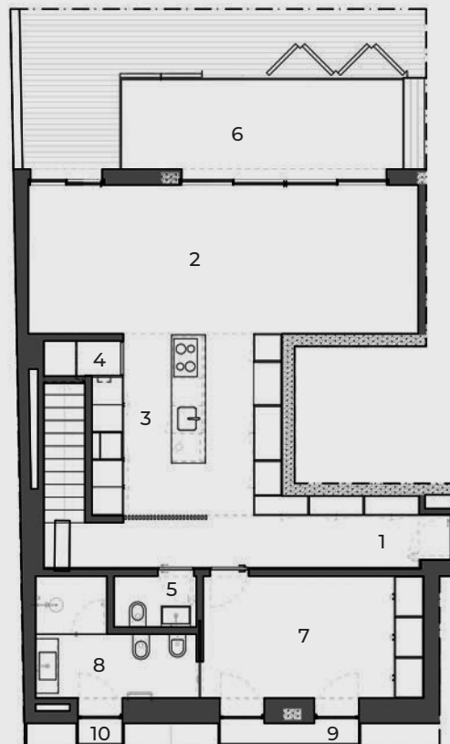
PISO 3
